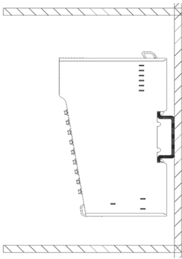
①水平安装侧视图
