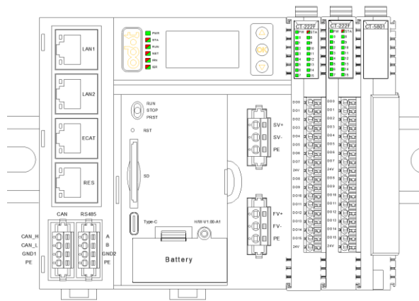
②水平安装
